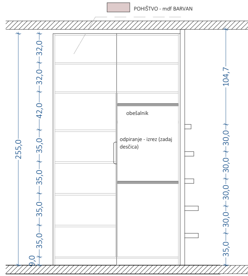
naris
