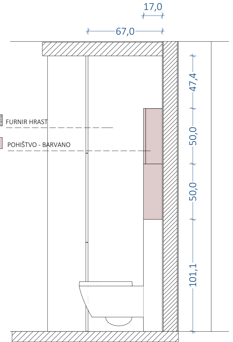
stranski ris
