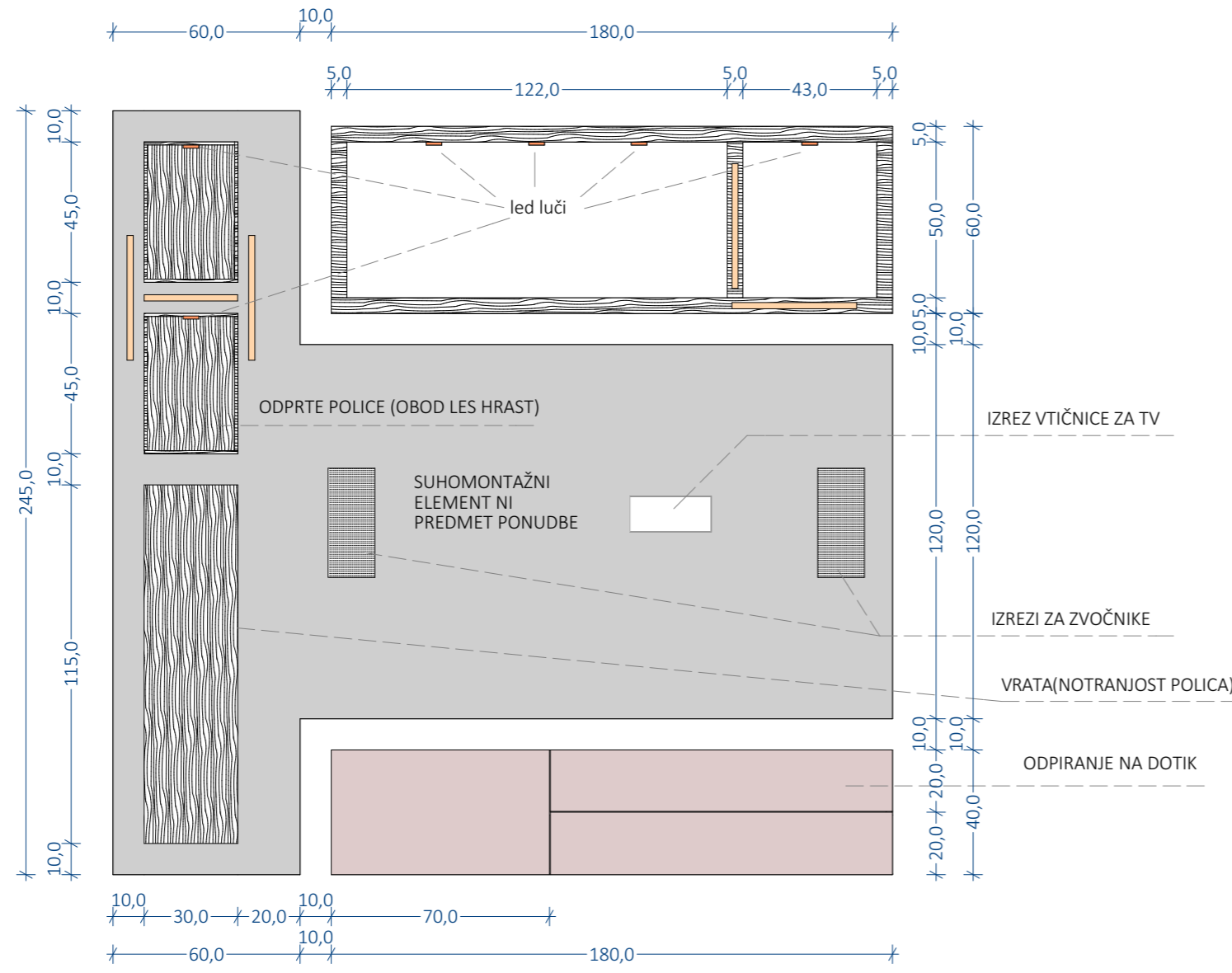
NARIS
