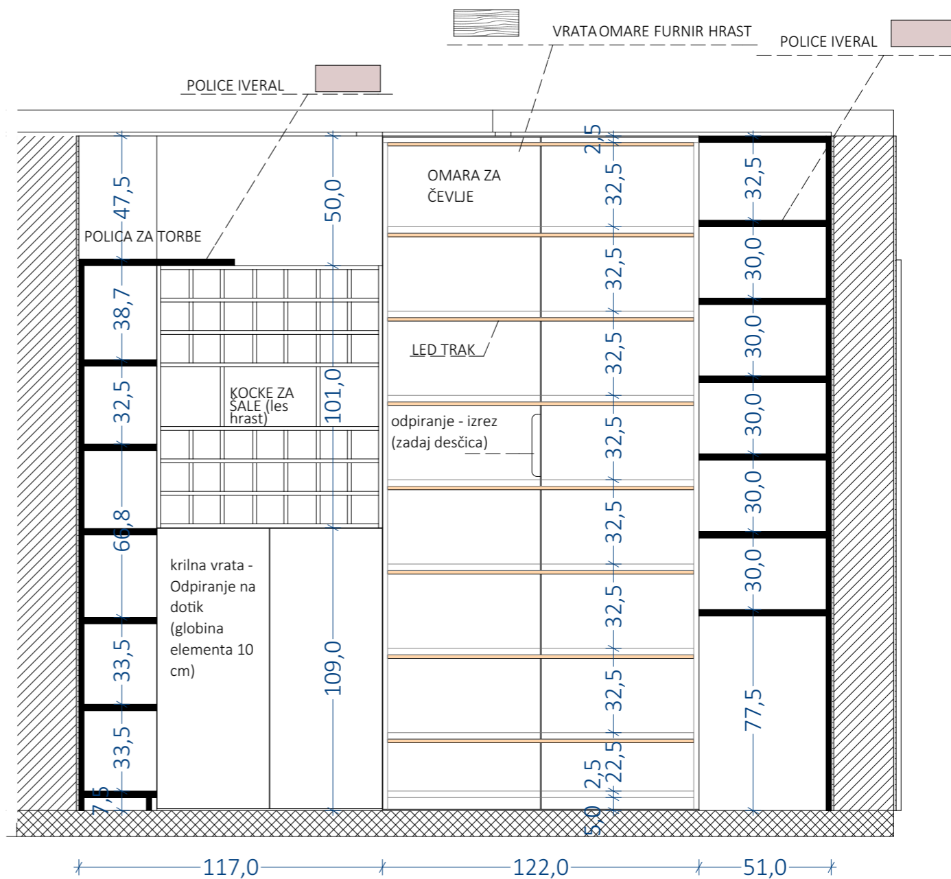
pogled B
