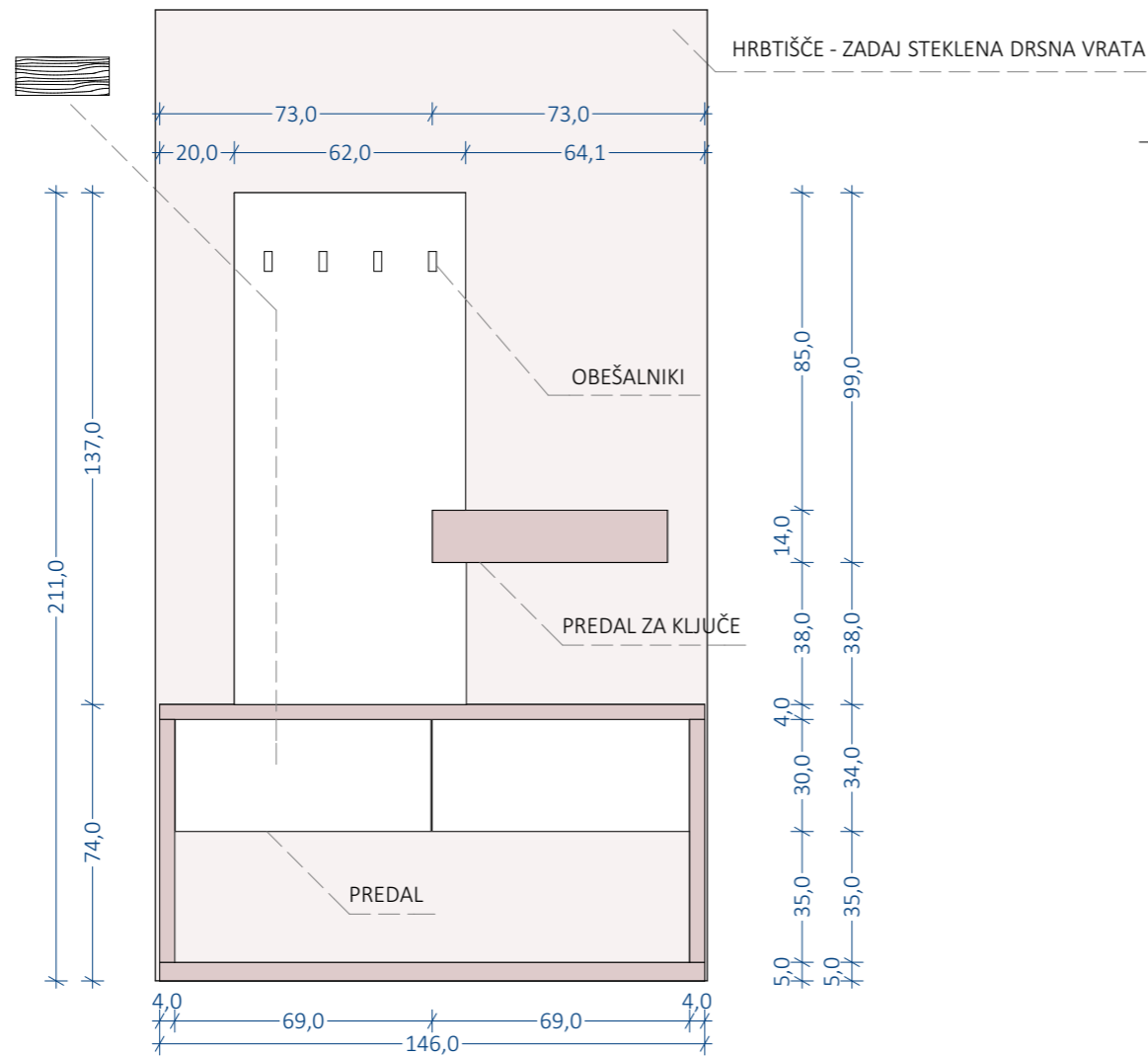
NARIS
