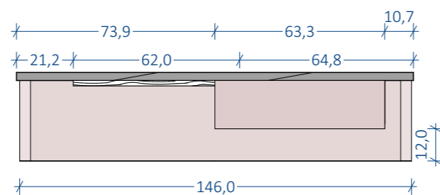
TLORIS
