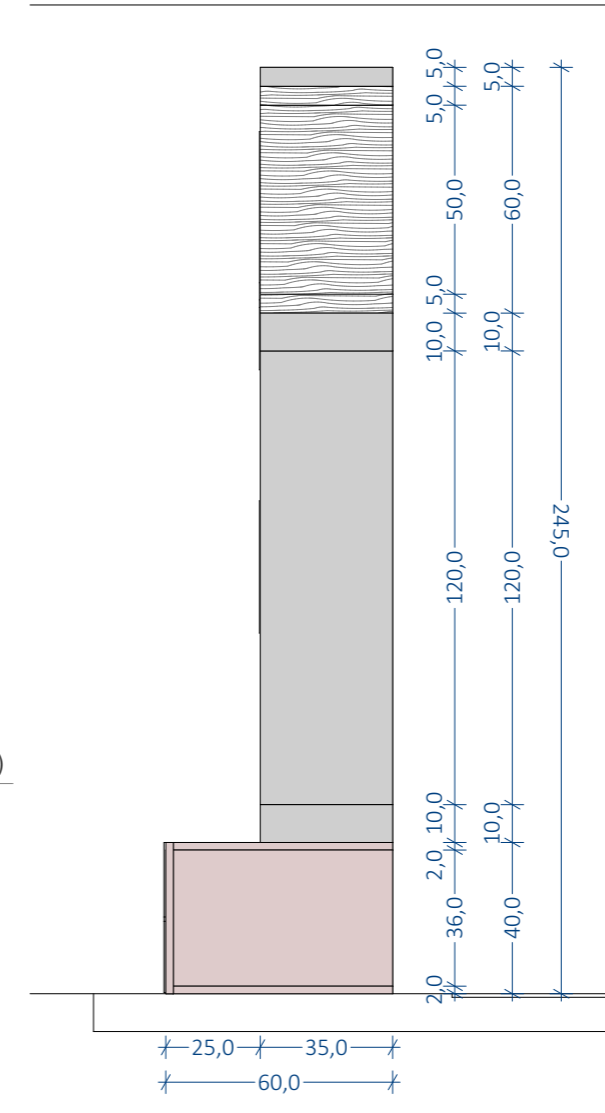
STRANSKI RIS
