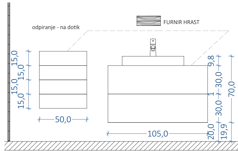
naris
