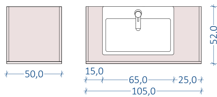
tloris
