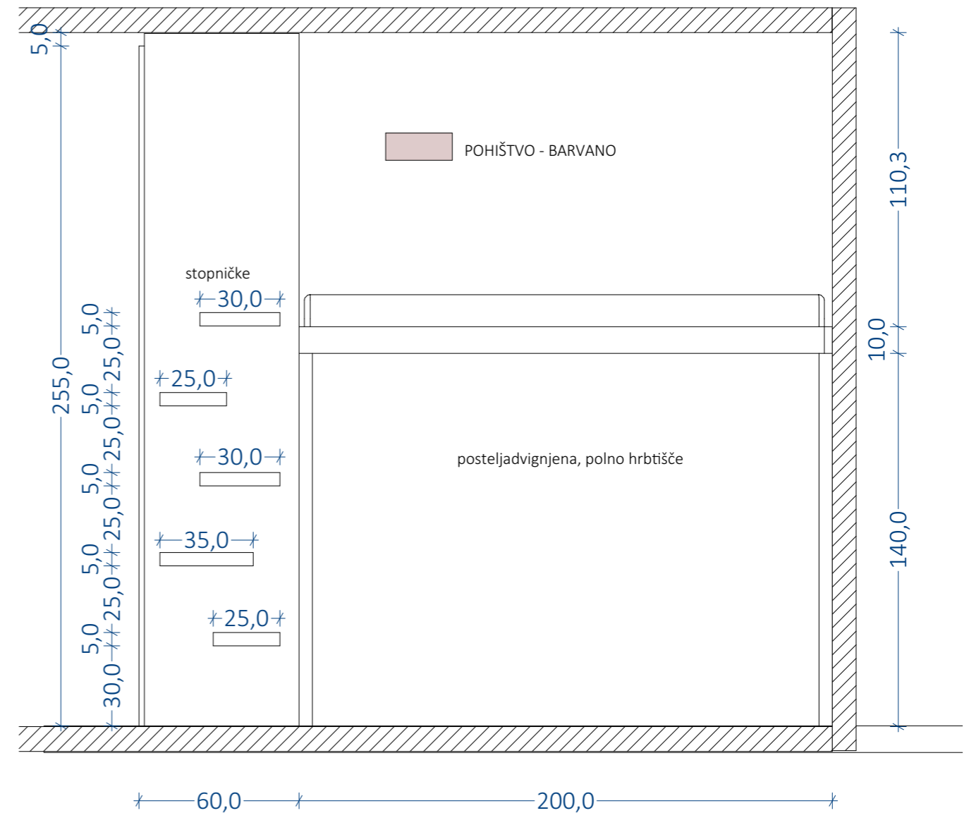
stranski ris
