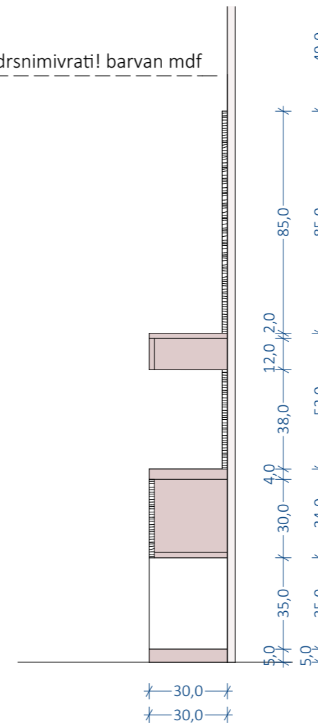
STRANSKI RIS
