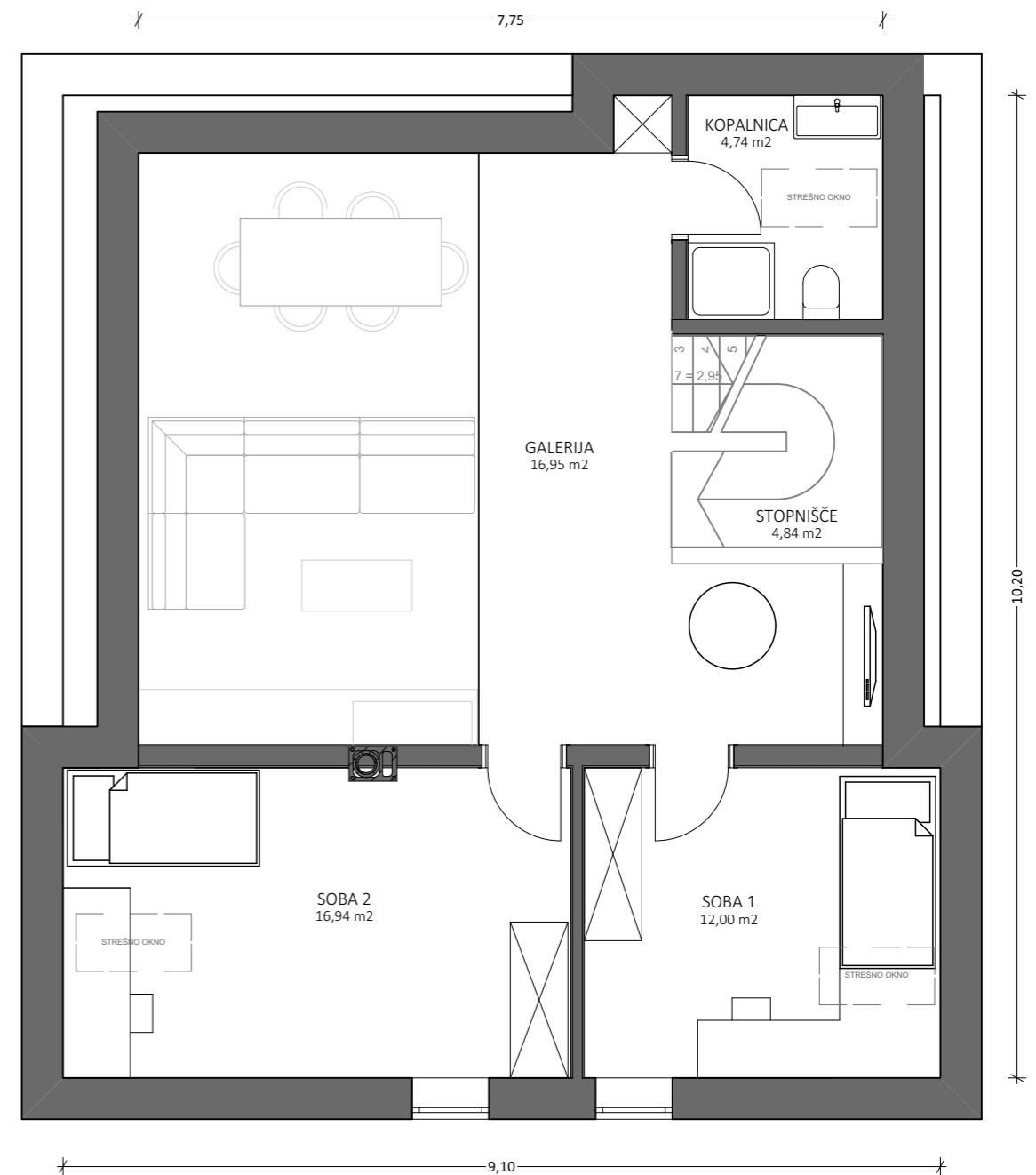
TLORIS NADSTROPJA
