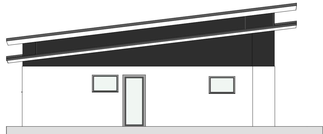
MIJA FASADA 4 1:100
