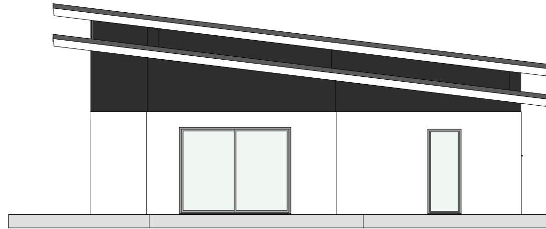
MIJA FASADA 3 1:100
