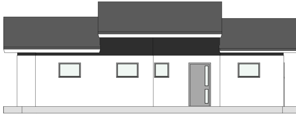
MIJA FASADA 1 1:100
