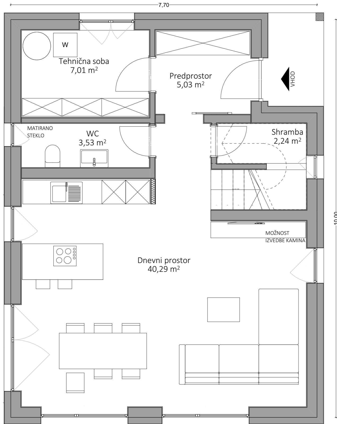
PRITLIČJE
